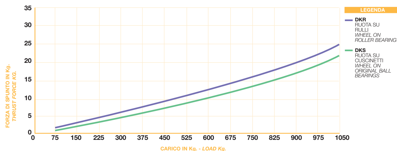
TEST EFFETTUATO SU UN CARRELLO DOTATO DI 4 RUOTE IN POLIURETANO Ø 160 TEST EFFECTED ON A TROLLEY EQUIPPED WITH 4 POLYURETHANE CASTORS Ø 160
