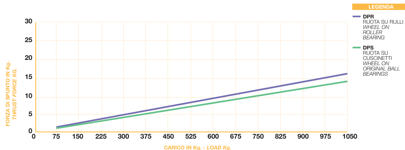
TEST EFFETTUATO SU UN CARRELLO DOTATO DI 4 RUOTE IN POLIURETANO Ø 160 TEST EFFECTED ON A TROLLEY EQUIPPED WITH 4 POLYURETHANE CASTORS Ø 160
